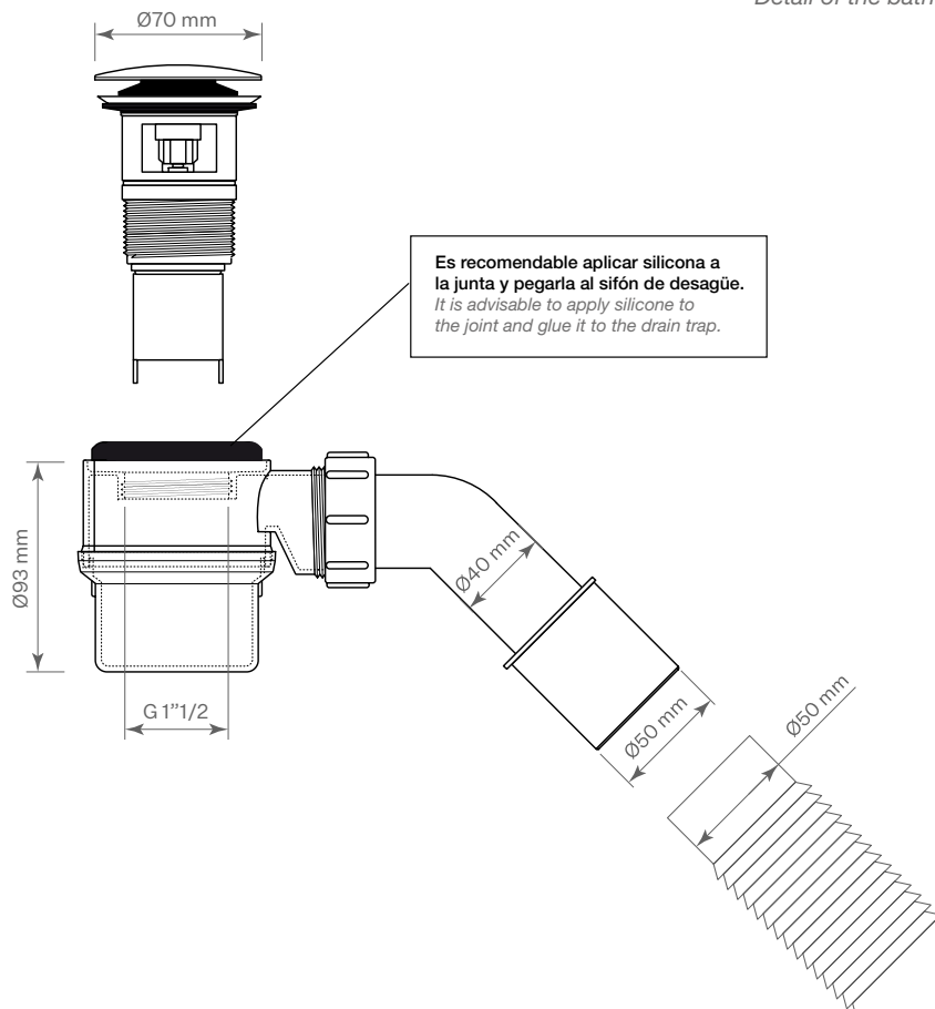
Detalle de la válvula y sifón de la bañera. Detail of the bathtub valve and siphon.
