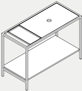
120×55×H80 cm STP 120 01
