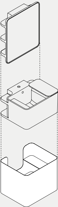
59,5×49,5×H50,5 cm ANF CES Cesta porta biancheria Anfibia in alluminio verniciato bianco opaco. Anfibia white matt painted aluminium laundry basket.
