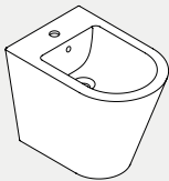
54×37×H42 cm FMBIT000000M Bidet terra monoforo. One hole floor standing bidet.
