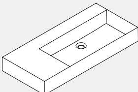
102×46×H12,5 cm ELLP10246LQ0
