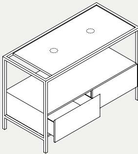
120×55×H80 cm STA 120 04
