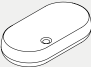
75×40×H16 cm NULA07540000 Lavabo da appoggio. Over-counter washbasin.
