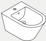
54×37×H34 cm FMBKS000000M Bidet sospeso monoforo. One hole wall hung bidet.
