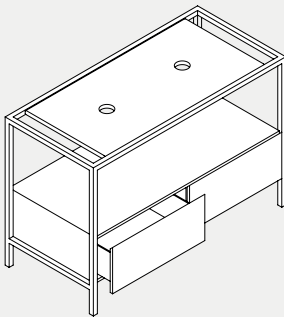
120×55×H80 cm STA 120 03
